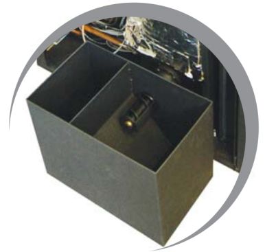
Kit estrazione cenere su braciere e scambiatore fumi, con motoriduttore e serbatoio esterno rimovibile a due vani.
